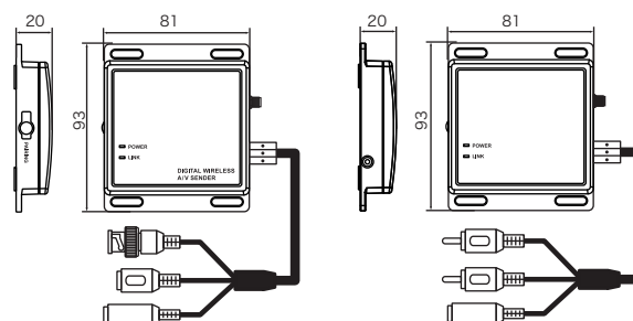
AG808T(送信機)
