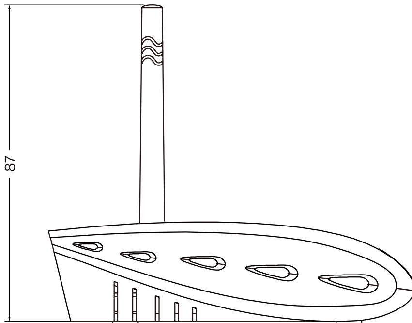
側面
