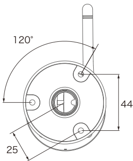
ブラケットベース
